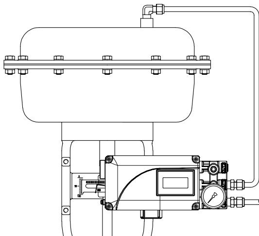
图4-1：单作用直行程执行器
