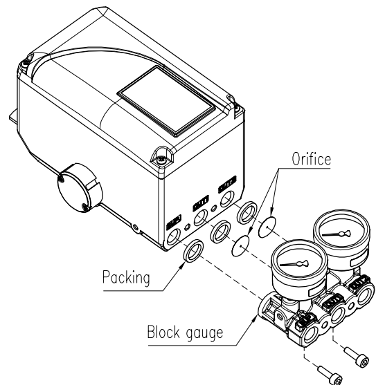
图6-1: 板型孔口件安装
