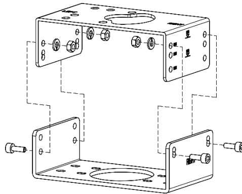
图3-12: 支架分解图
