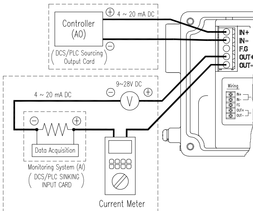
图9-3: 设置发送器
